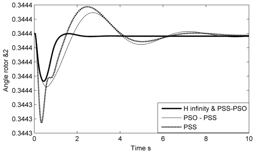
Fig. 3: Angle rotor \delta_2
