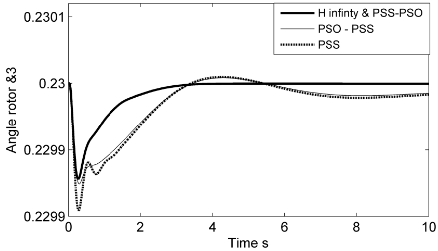
Fig. 4: Angle rotor \delta_3
