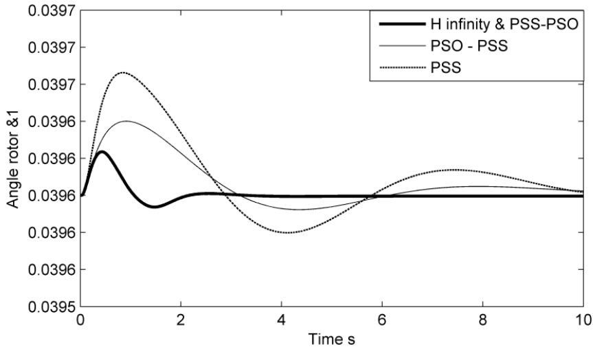
Fig. 2: Angle rotor \delta_1
